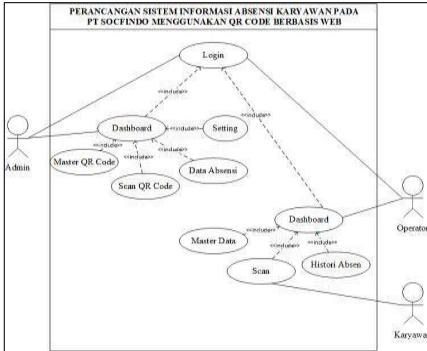
Gambar 2. UML Perancangan Sistem Informasi Absensi PT. SOCFINDO Berbasis QR Code Berbasis Web.
