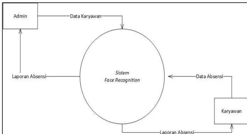
Gambar 1. Data Flow sistem absensi yang sedang berjalan pada PT.SOCFINDO
