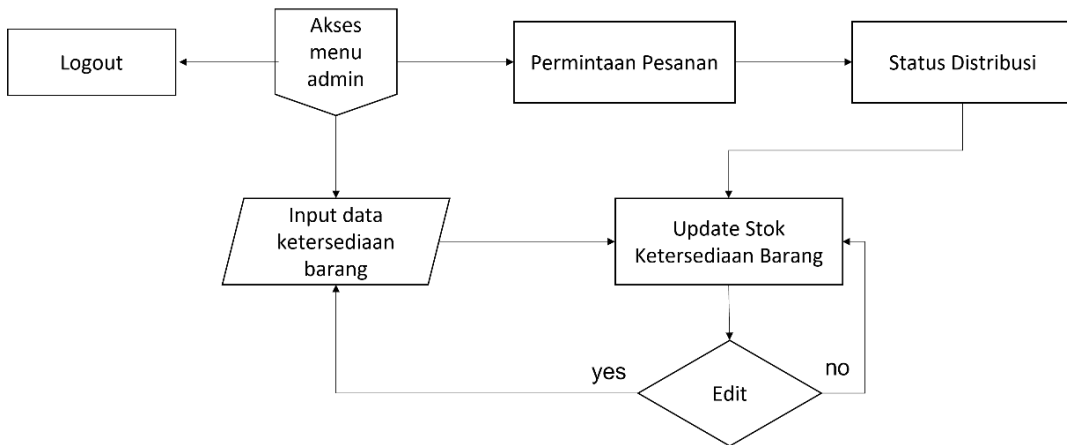
Gambar 4. Flowchart Perancangan Sistem Tampilan Utama
